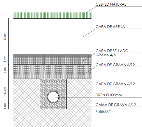
DETALLE DEL PAQUETE DE CONSTRUCCIÓN . escala.: 1/10
